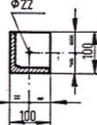
PREREZ „D-D“
