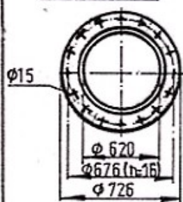
POGLED „B“
