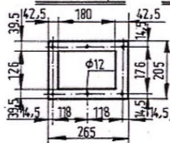
POGLED „C“
