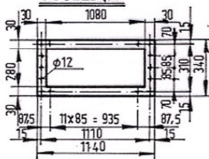
POGLED „A“
